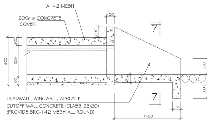
LONGITUDINAL SECTION SCALE 1:25
