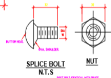
NUT N.T.S
