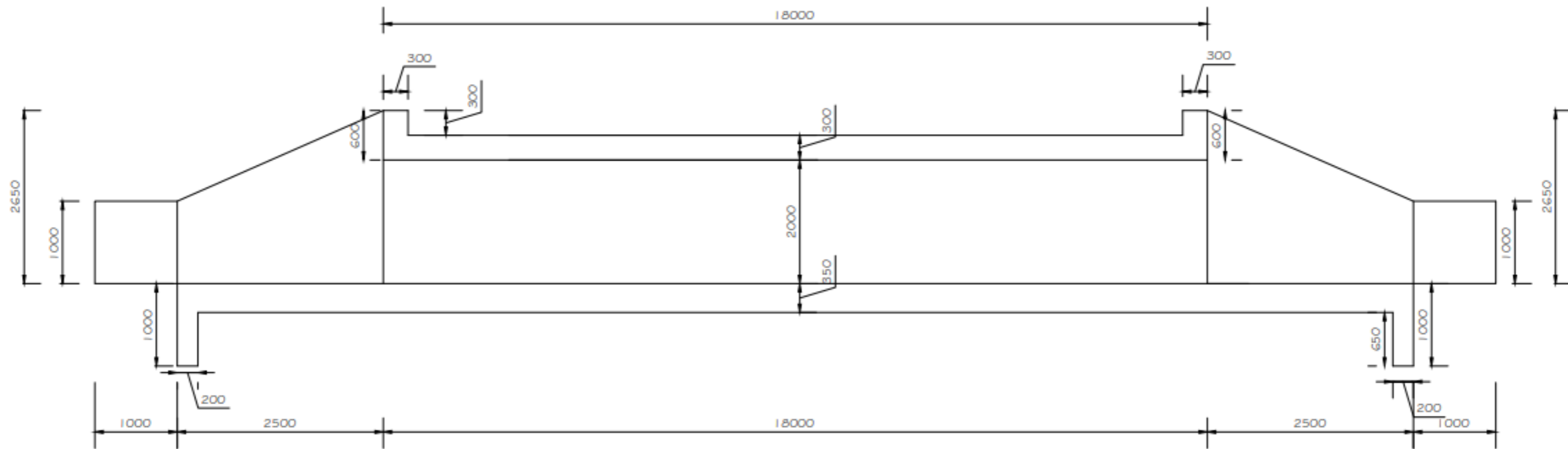
SECTION A-A
