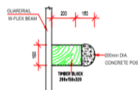
SECTION A-A SCALE:- 1:10
